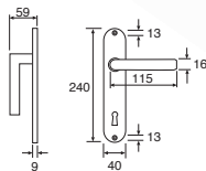
Art. 00250 MANIGLIA CON PLACCA Handle with plate
